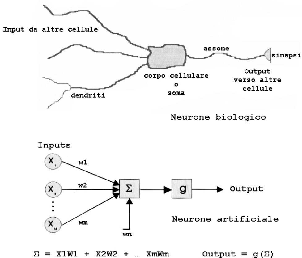
Fig 3-2: Modello di un neurone biologico e di un neurone artificiale ad una uscita. La "g" è detta funzione logistica di attivazione.
