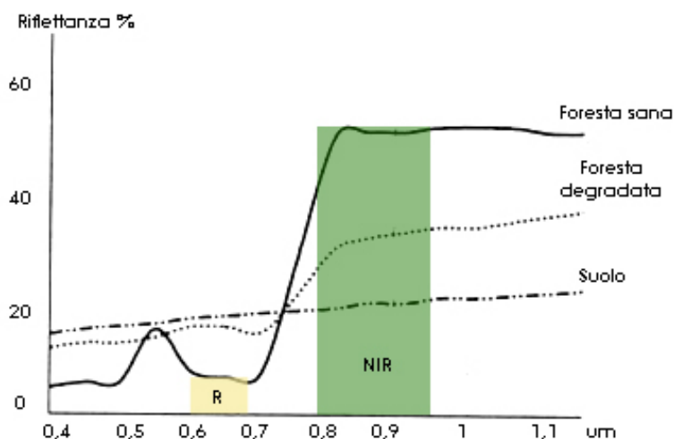
Fig 4-19: Contrasto spettrale della vegetazione sana fra la banda Rosso e la banda infrarosso prossimo NIR.
