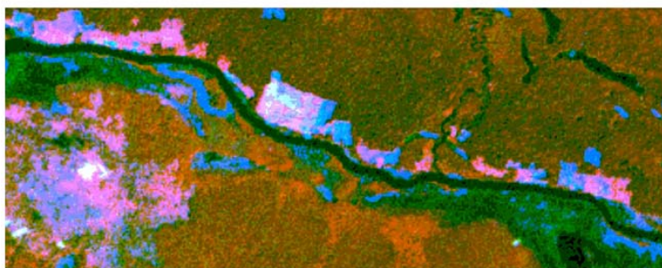
CC con OIF maggiore: TM 417 RGB 1992. Zoom su Rio San Pedro
